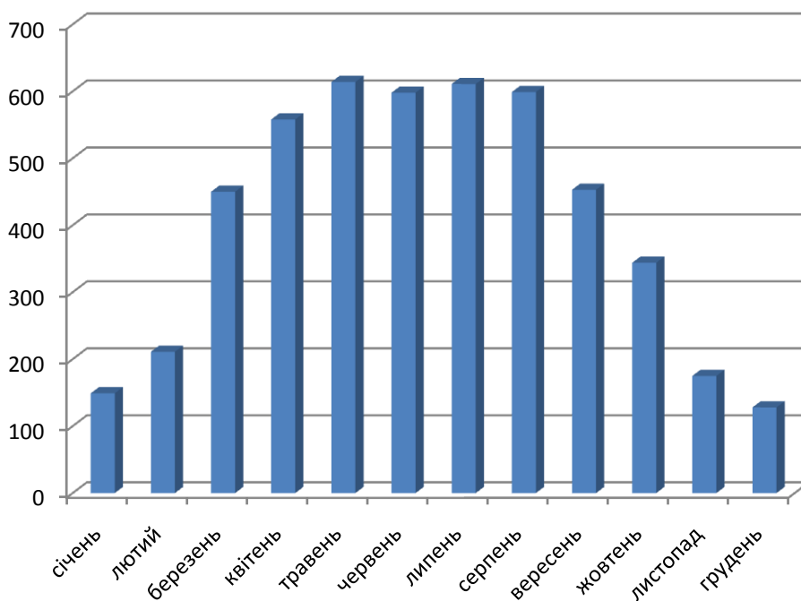
Генерація електроенергії сонячною станцією потужністю 5 кВт протягом року (енерговиробіток кВт · год по місяцях)
